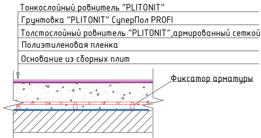
Сечение готового покрытия тонкослойного ровнителя.
